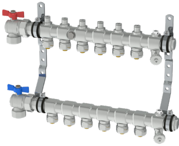
Teollisuusjakotukki
