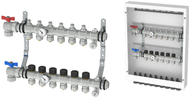
Jakotukki
