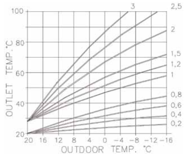
Figur 6. Värmekurvor.
