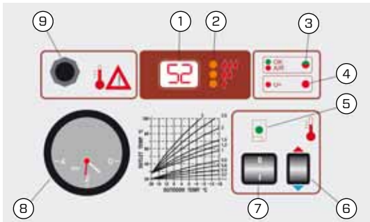
Figur 5. Elpannans manöverpanel.
