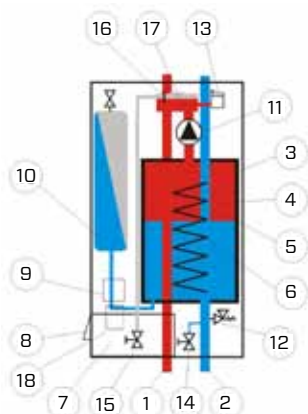
Figur 1. Elpannans ingående komponenter.
